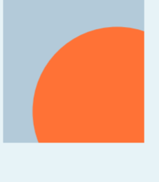
source-atop
